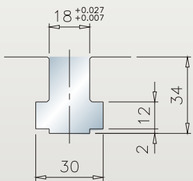
MV-800 T-slot dimensions
